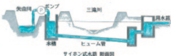
サイホン式水路 断面図
