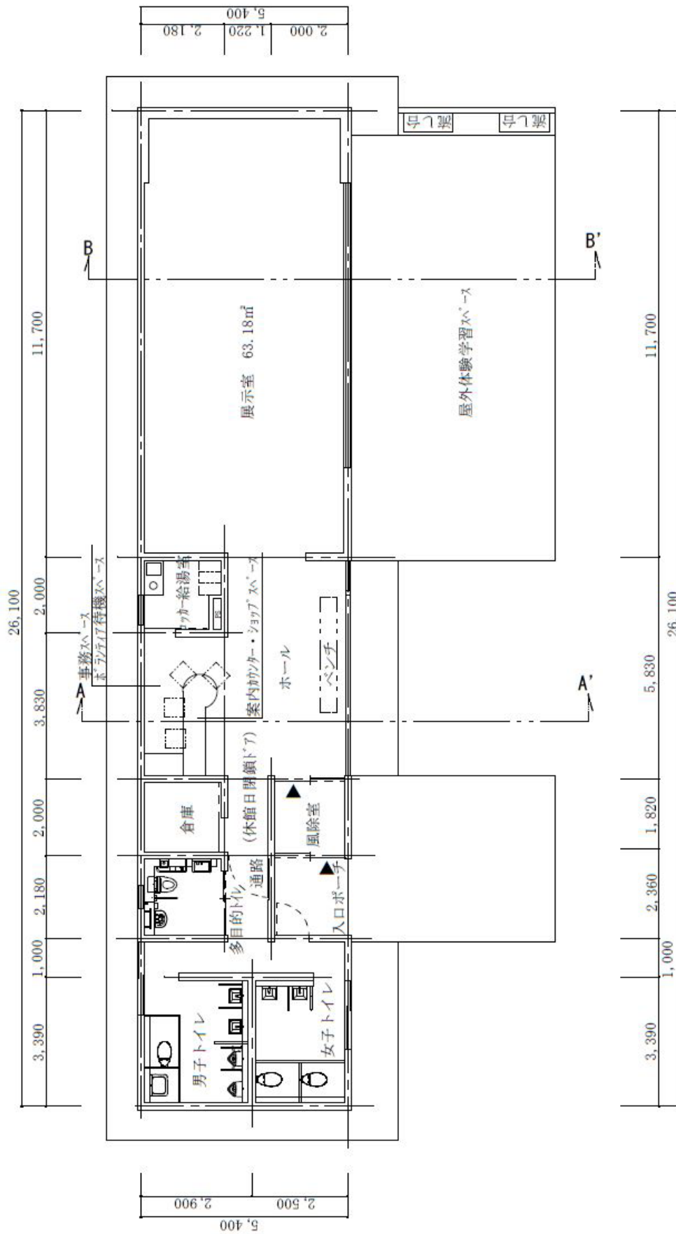
ガイダンス施設概要図
