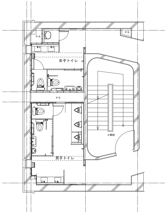
4～11階トイレ平面詳細図
