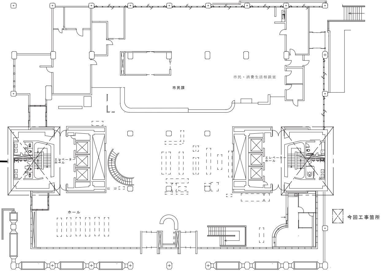
市庁舎1階平面図
