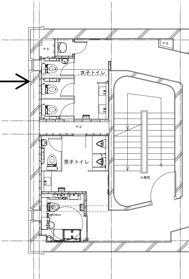
1～3階トイレ平面詳細図
