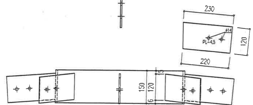
圓板センター金物
