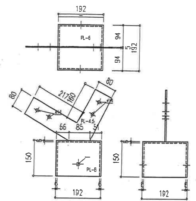
柱頭キャップ (方杖付き)
