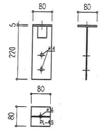
方杖T形金物
