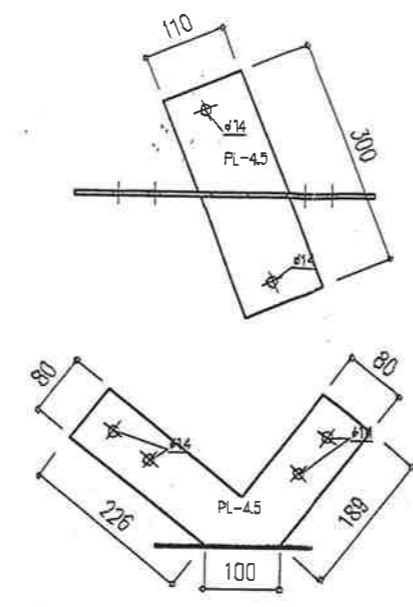
方杖T形金物
