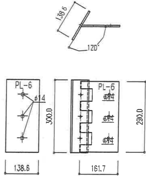
梁金物
