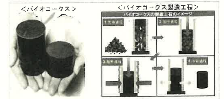
資料：神戸市のバイオコークス製造工程
