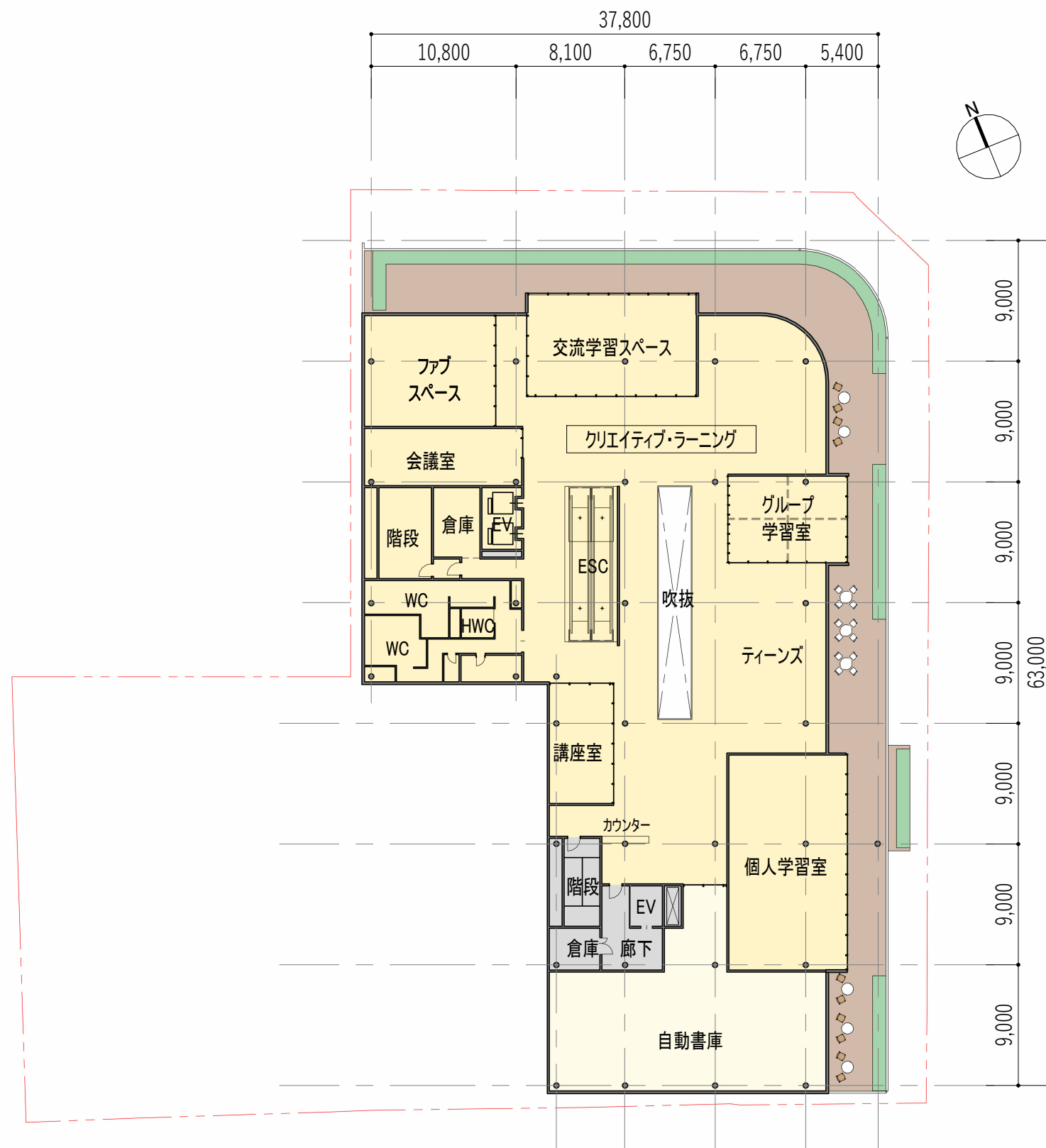
6階平面図 (1:400)
